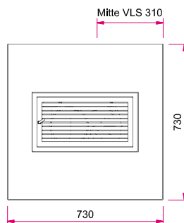
Draufsicht M 1:25
