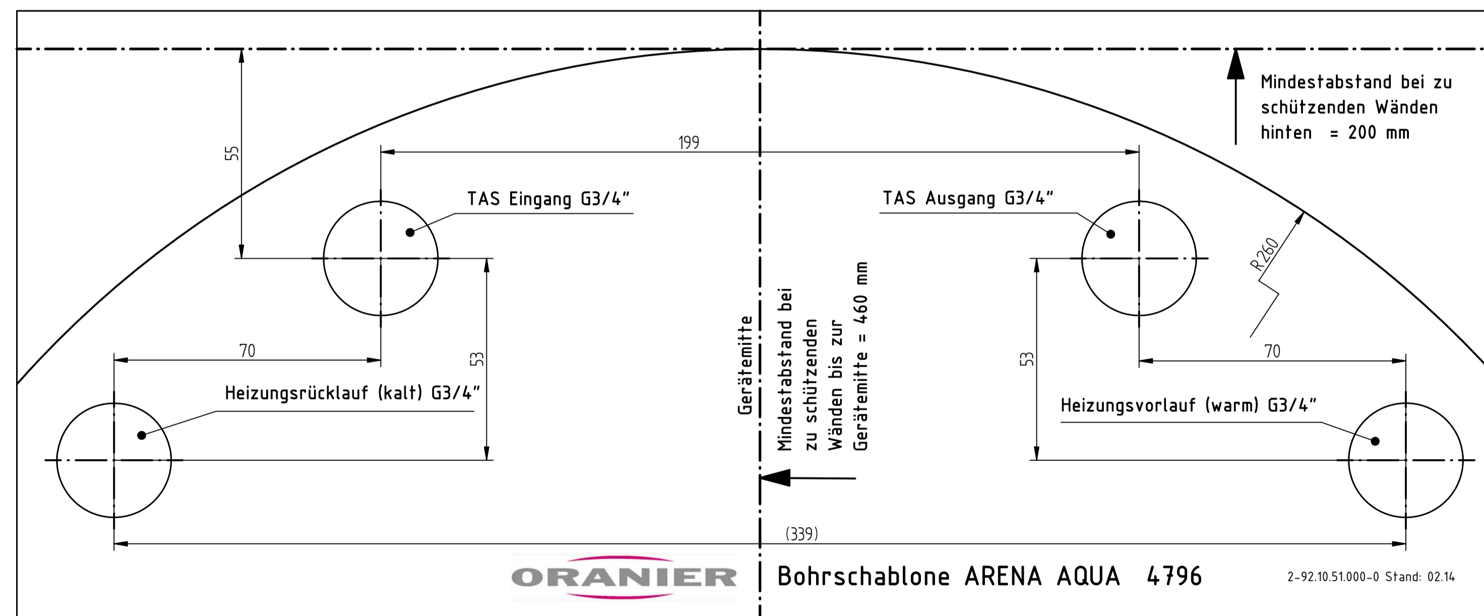
Darstellung der bedruckten Schablone
