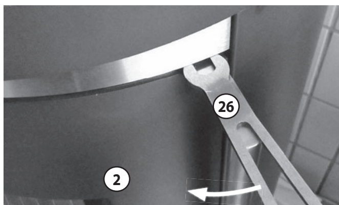
Brennerschale vor...
