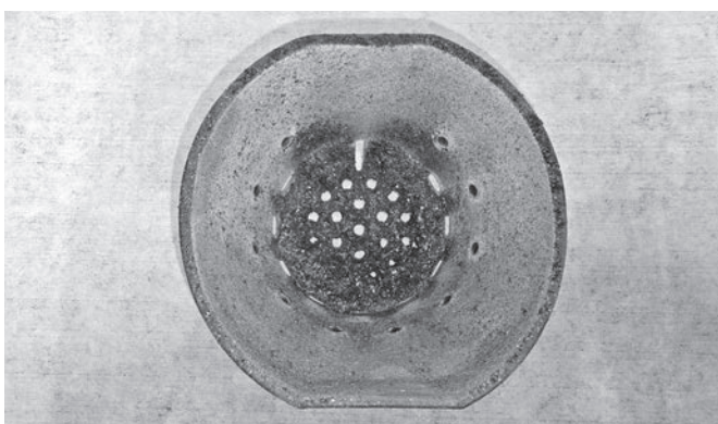
Brennerschale (5) vor...
