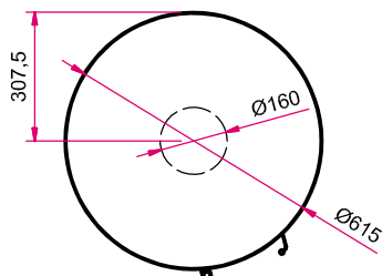
Draufsicht M 1:20
