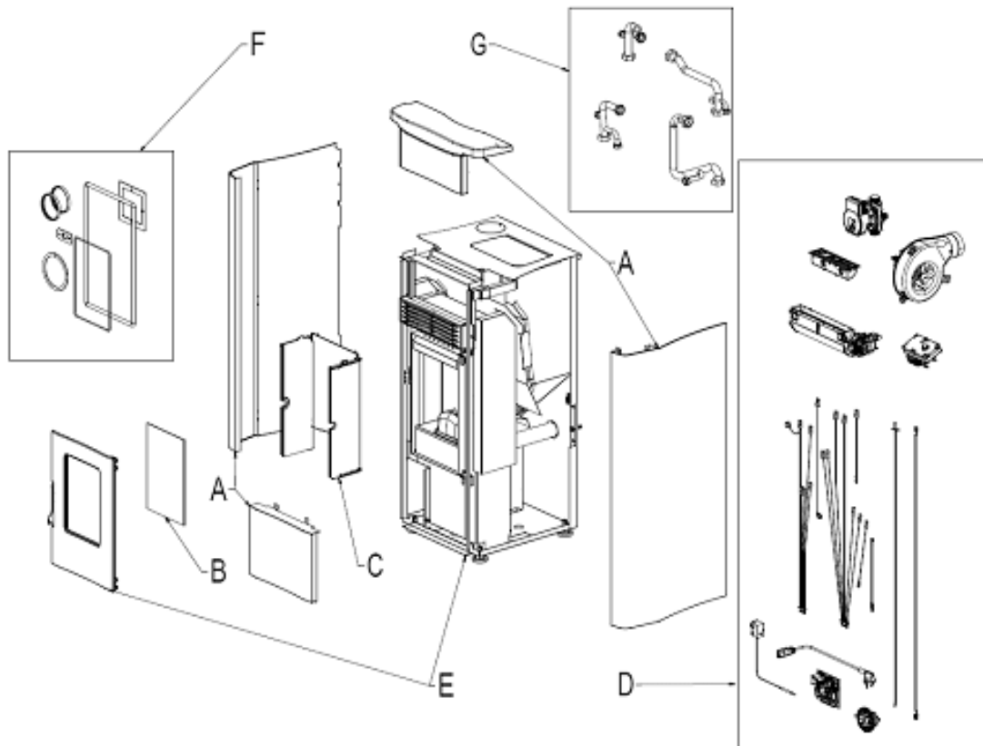
Fig. 1 - Explosionszeichnung
