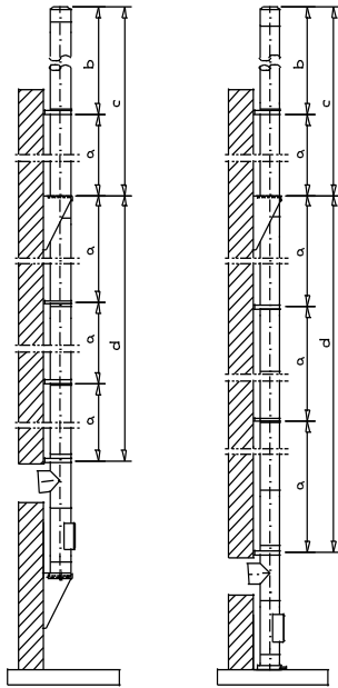
Bild 1: Aufbauhöhen
