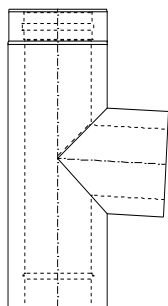
T-Anschluss 87°
