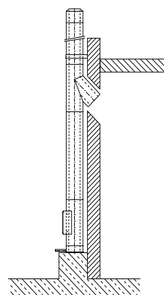
Bild 7: Aufbau mit Grundplatte für Sockelmontage
