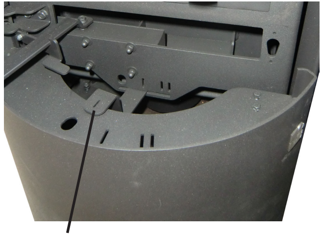
Bedienhebel für die Verbrennungsluftzufuhr
