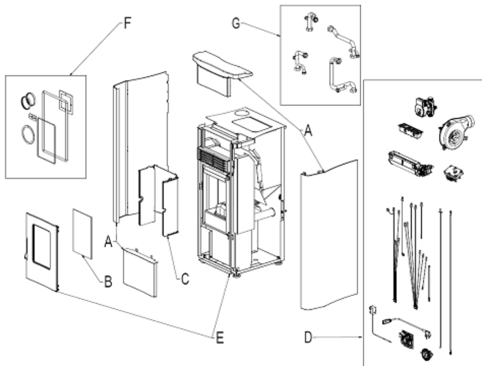
Fig. 1 - Explosionszeichnung
